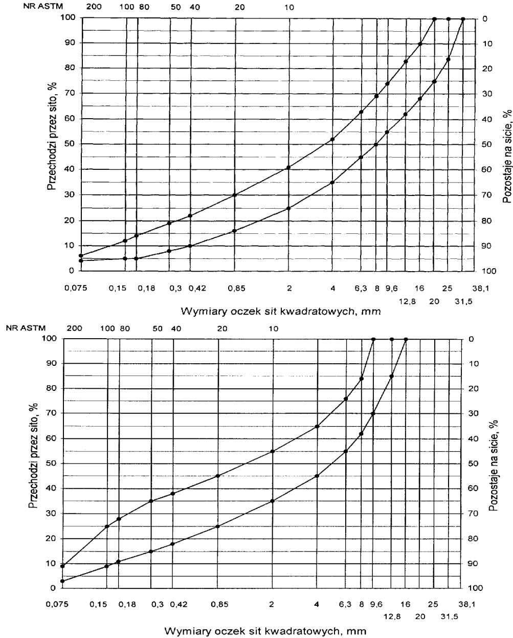
Rys. 6. Krzywe graniczne uziarnienia mieszanki mineralnej BA od 0 do 12,8 mm do warstwy wiążącej, wyrównawczej i wzmacniającej nawierzchni drogi o obciążeniu ruchem KR1 lub KR2
