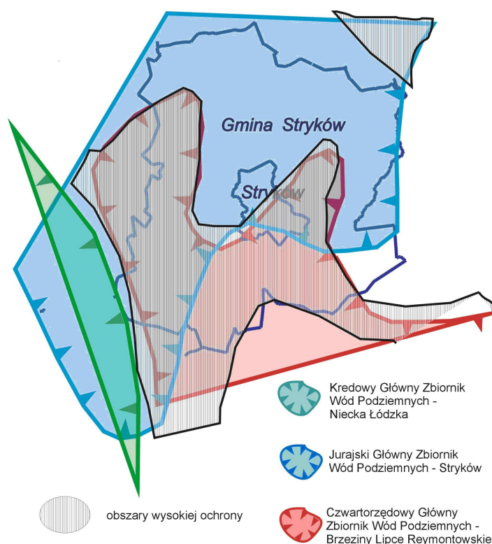
Rysunek 8. Główne zbiorniki wód podziemnych występujące na terenie Miasta - Gminy Stryków
