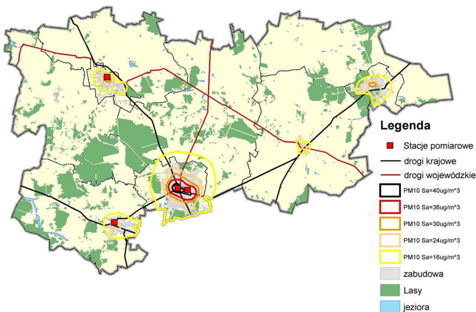
Rysunek 6. Średnie roczne stężenie pyłu PM10 w powiecie zgierskim w 2007 r.
