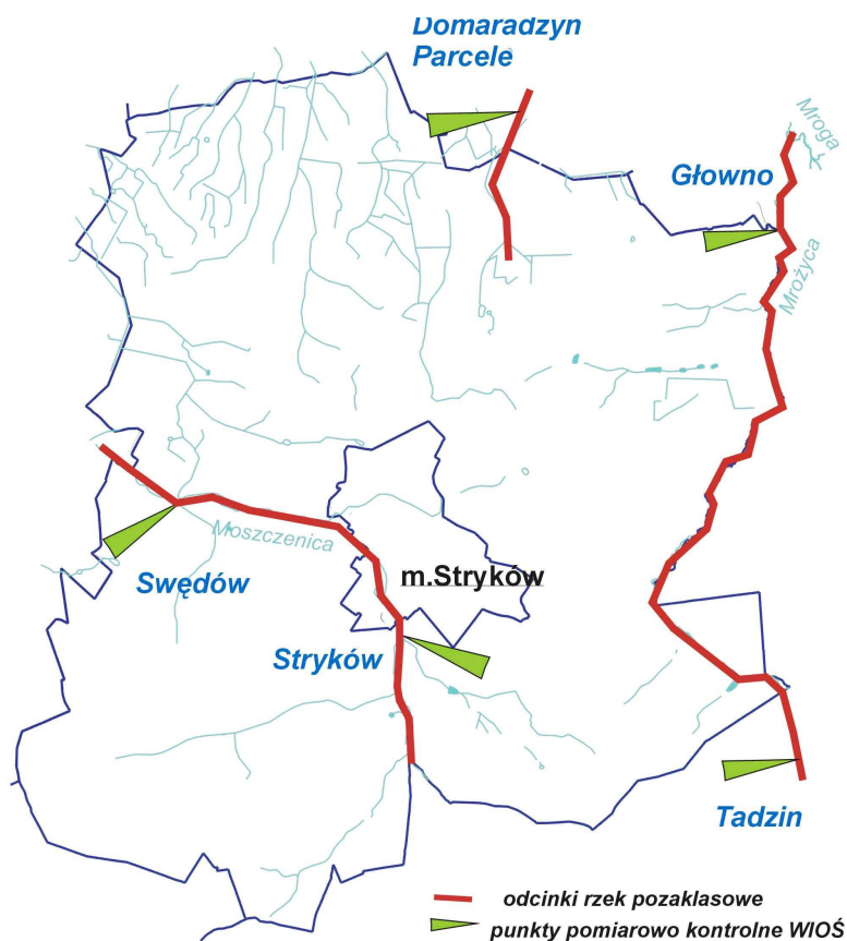
Rysunek 7. Jakość wód powierzchniowych w Mieście Gminie Stryków oraz punkty pomiarowo kontrolne WIOŚ
