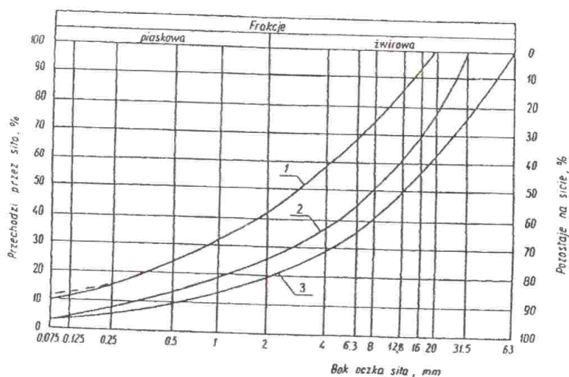
Rys. 1. Pole dobrego uziarnienia kruszyw dla podbudowy
